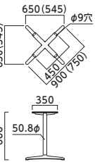
GF-PO-S 550L・ 650L・750L・900L (研磨仕上げ)
