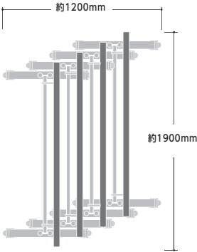
スタック収納時スペース (天板サイズ 1800W 900D)
